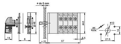
Zmiana liczby obrotów - Rozłącznik w układzie Dahlandera (2biegi O-D-YY)
