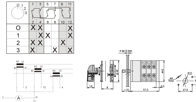
Schemat amperomierzowy
