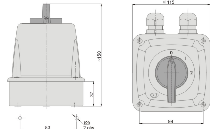
max. liczba segmentów-4 z dławnicami PG16
