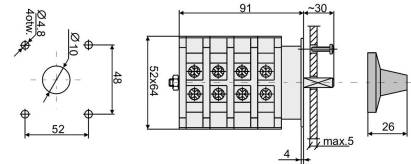
Zmiana liczby obrotów - Rozłącznik w układzie Dahlandera (2biegi O-D-YY)
