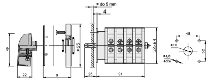
Zmiana liczby obrotów - Rozłącznik w układzie Dahlandera (2biegi O-D-YY)
