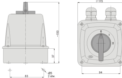
max. liczba segmentów-4 z dławicami PG16
