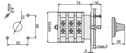
Zmiana liczby obrotów - Rozłącznik w układzie Dahlandera (2biegi O-D-YY)
