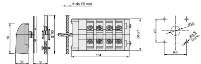
Zmiana liczby obrotów - Rozłącznik w układzie Dahlandera (2biegi O-D-YY)
