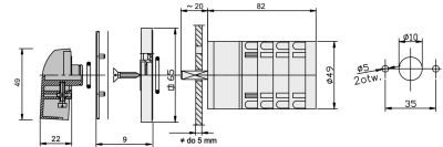
Zmiana liczby obrotów - Rozłącznik w układzie Dahlandera (2biegi O-D-YY)
